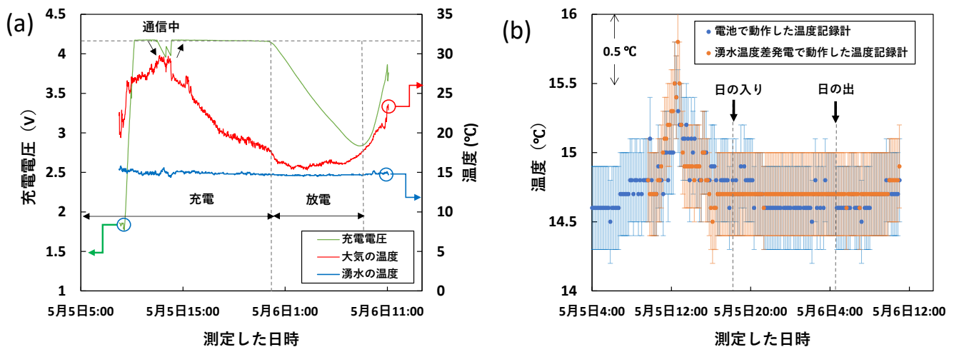
図4 (a) 熱電モジュールからキャパシターに充電される様子。充電試験を行った当日（2022年5月5日）の湧水と大気のも同じグラフ内の第二軸に示した。(b)湧水温度差発電装置で駆動した温度記録計で計測した湧水の温度。参考に、電池で駆動した温度記録計で計測した湧水の温度も示した。
