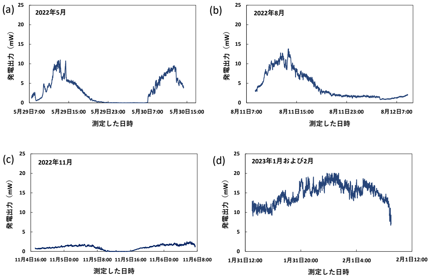
図3 湧水温度差発電から得られる電力の季節変動 (a) 2022年5月 (b) 2022年8月 (c)2022年11月 (d)2023年1月および2月
