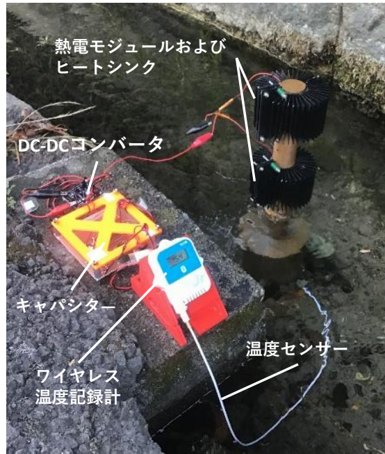
図2 湧水と大気の温度差が生み出す電力を温度記録計へ供給し、水路を流れる湧水の温度を計測している様子
