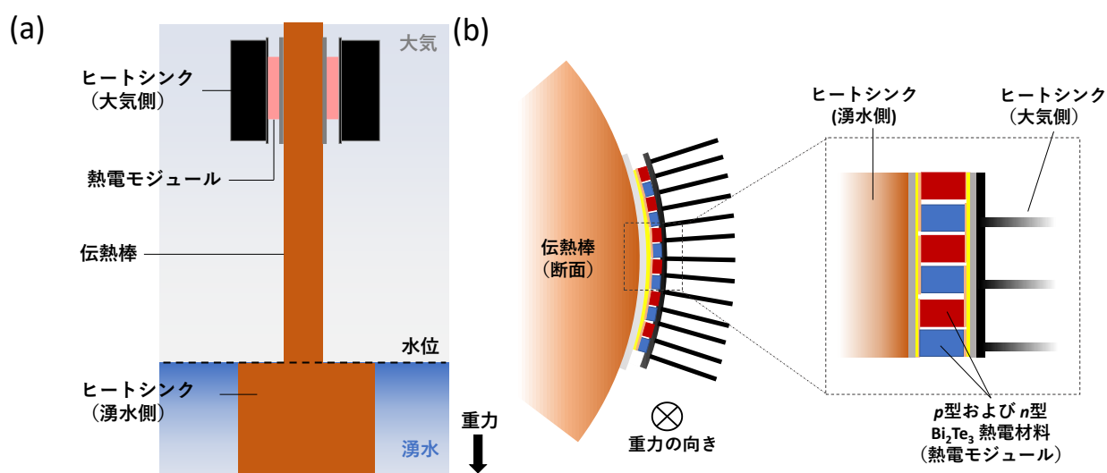
図 1 (a) 開発した湧水温度差発電装置 (b) 湧水温度差発電装置を上方から眺めた断面図と拡大図
