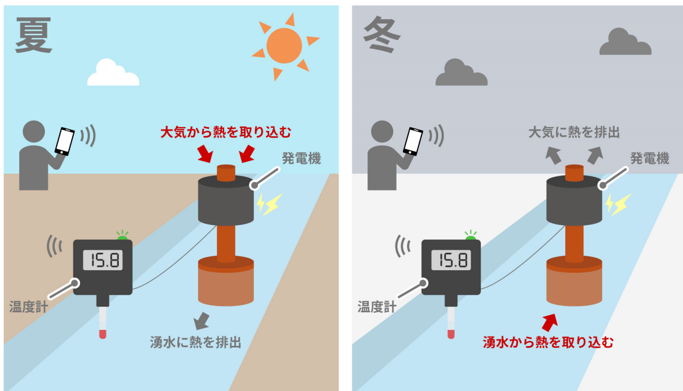
湧水温度差発電の原理図
